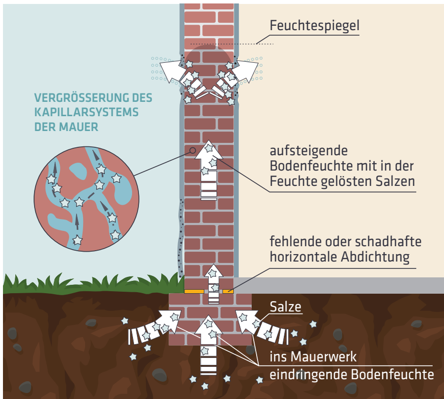
Grafik 1: Aufsteigende Bodenfeuchte, mittransportierte baustoffschädigende Bodensalze
